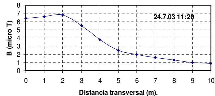
Campo magnético de los cables subterráneos de MT
